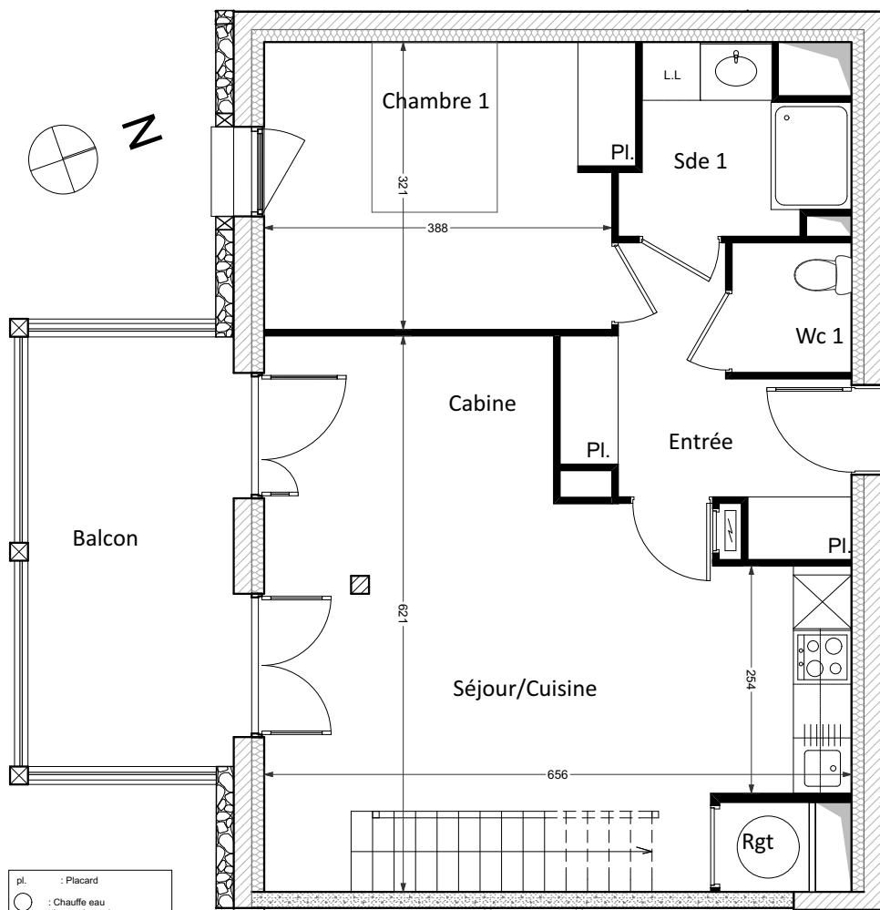
Niveau 1
