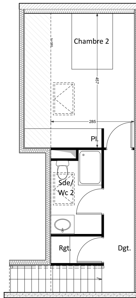
Niveau 2
